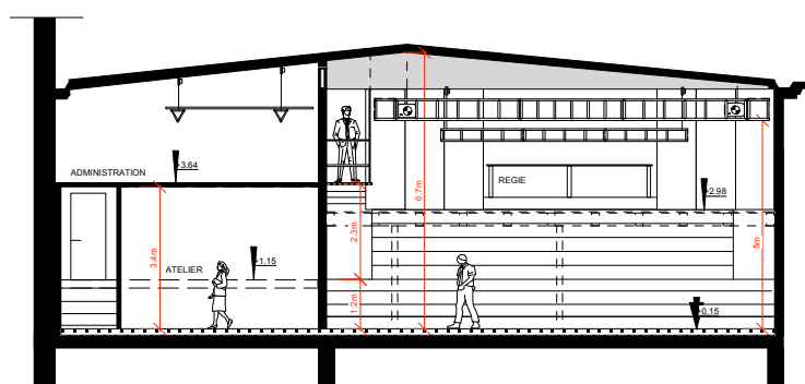
Coupe B_B
