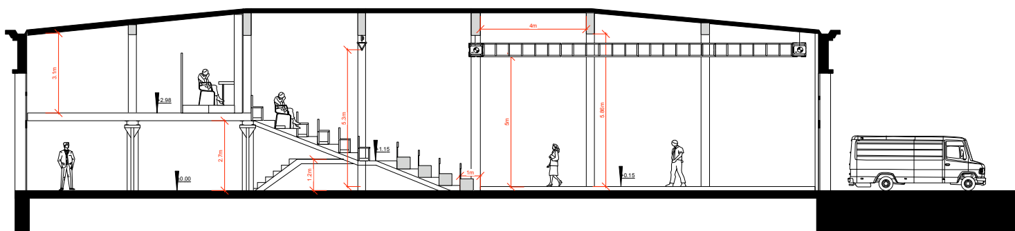
Coupe A_A
